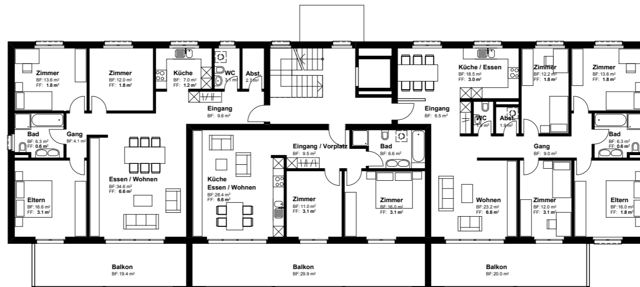
1./2. Obergeschoss
